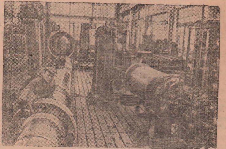
Довбасс Орден Ленина Ново-Краматорский машиностроительный завод имени Сталина выпускает подъемные машины для восстанавливаемых шахт Юга. На снимке: обработка агрегатов шахтоподъемной машины в цехе № 1. Фото С. Нордштейна. Фотохроника ТАСС
