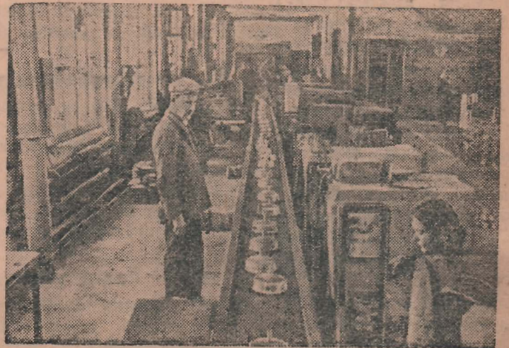
Тульский завод, где директором тов. Орловский, ваною реконструирован и снабжен новейшим оборудованием цех ширпотреба. Установлен конвейер. На снимке: примусы на конвейере. Фото В. Лисовкина.
