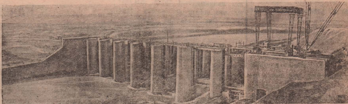
Заканчивается сооружение плотины самой крупной в Узбекской ССР Фархадской гидроэлектростанции на реке Сыр-Дарья. На снимке: общий вид плотины Фархадской ГЭС. Фото С. Бессонова.
