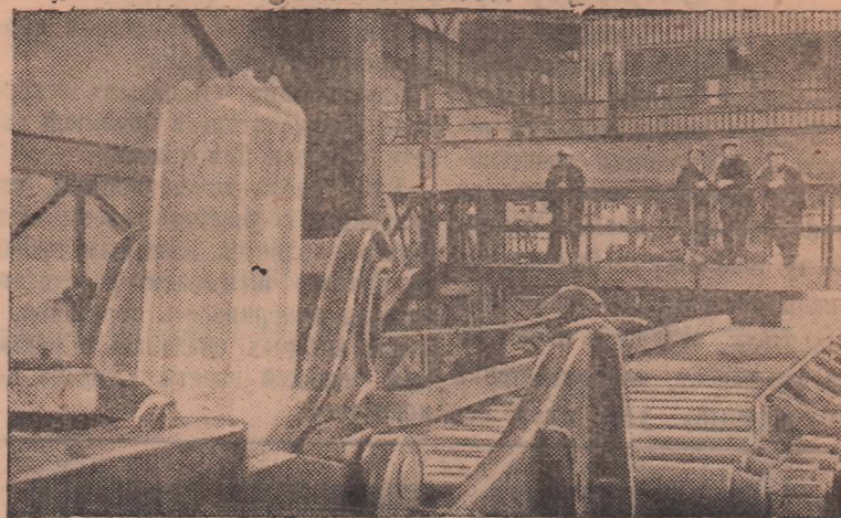
Магнитогорский металлургический комбинат. Подача 7-тонной чугушной чушки на рольганги блюминга. Фото А. Скурихина. Прессклише ТАСС
