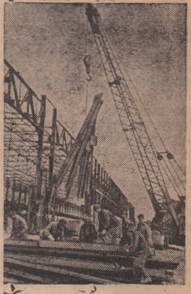
Мариуполь. На стройке прокатного цеха завода „Азовсталь“. Подъемный кран за установкой железных конструкций пролета строющегося рельсо-балочного стана. Фото П. Кашкеля. Прессклише ТАСС.
