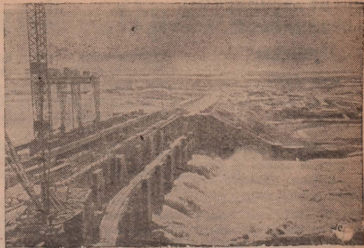
Узбекская ССР. Плотина Фархадской гидроэлектростанции — одной из крупнейших новостроек новой Сталинской пятилетки. Фото М. Гор. Прессклише ТАСС
