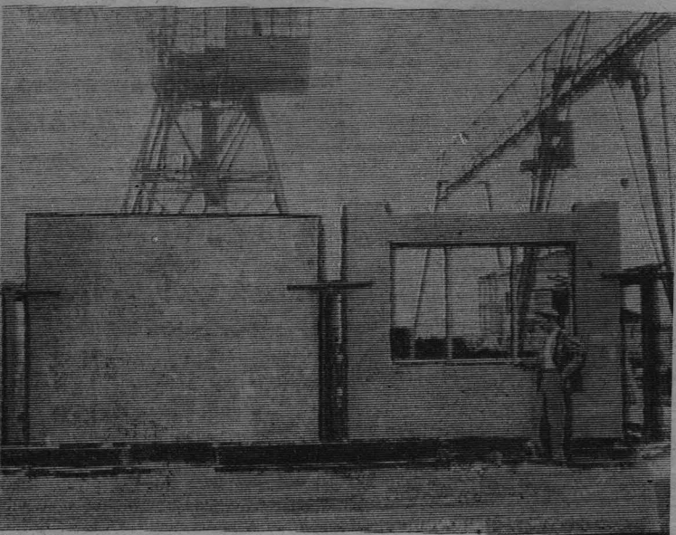
Готовые виброкирпичные панели
