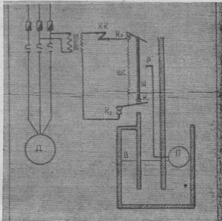
Принципиальная схема автоматической откачки воды насосом.
