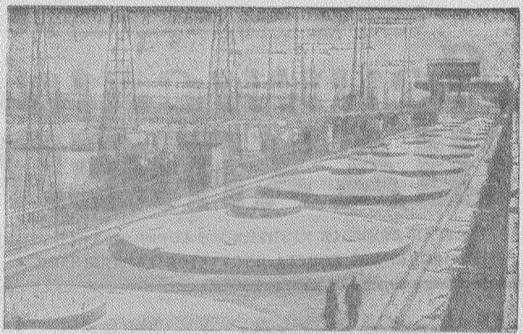
Кременчугская ГЭС. Ее мощность 625 тысяч киловатт. Это станция открытого типа, без здания машинного зала. Она уже выработала более 11/2 миллиардов киловатт-часов электроэнергии.
