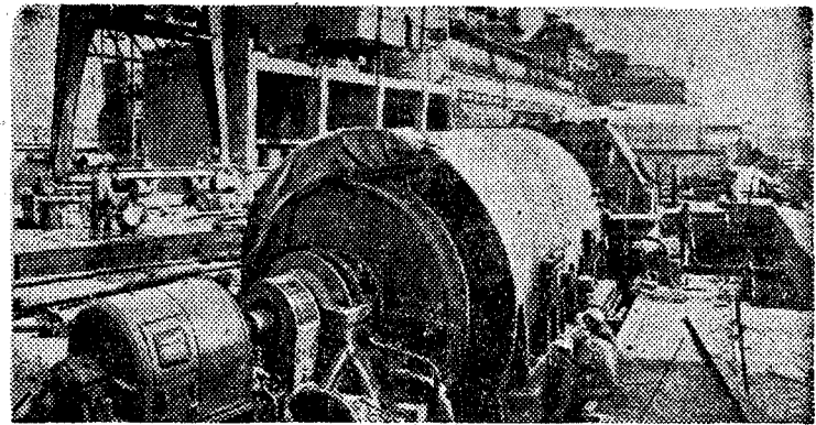
Душанбинская ТЭЦ — одна из крупных строек столицы Таджикистана. В эти дни здесь заканчивается монтаж нового энергоблока мощностью 50 тысяч киловатт. В дни юбилея Таджикистана агрегат даст ток.
