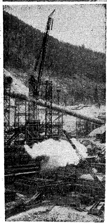
Красноярский край. Строители крупнейшей в мире Красноярской ГЭС готовят механизмы к началу больших бетонных работ, которые развернутся с нового, 1965 года по всему фронту строя. Идет монтаж мощных кабелькранов для укладки бетона в тело плотины. На снимке: правобережный котлован Красноярской ГЭС. Фотохроника ТАСС.
