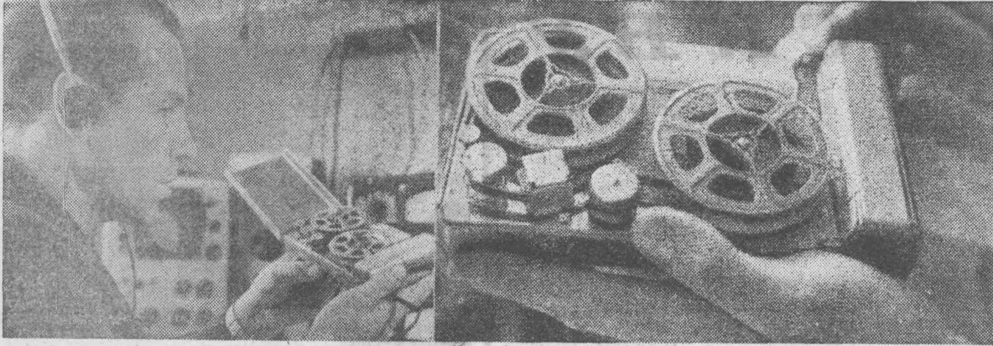
На Новосибирской областной радиовыставке в текущем году всеобщий интерес вызвал карманный магнитофон «Сигма». Этот миниатюрный аппарат, помещающийся на ладони, весит 400 граммов. Длительность записи на долгоиграющей пленке «Сигмы» составляет один час. На снимке: А. Н. Румянцев со своим карманным магнитофоном. Справа карманный магнитофон «Сигма». Фото В. Лещинского. Фдтохроника ТАСС.
