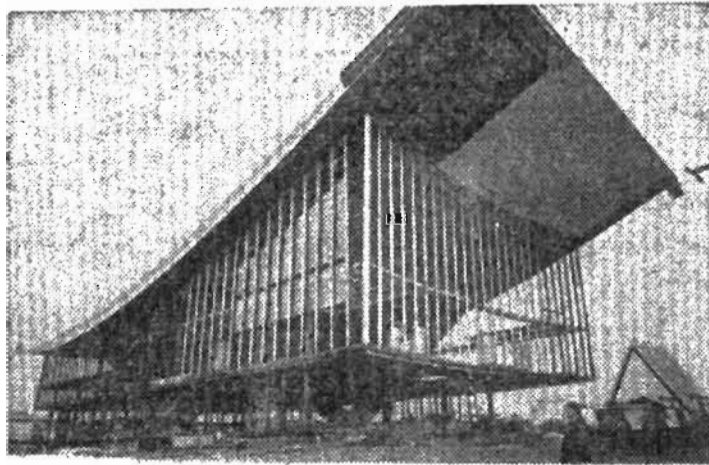
На снимке: строительство павильона СССР на Всемирной выставке в Монреале. Фото Ю. Королева. Фотохроника ТАСС.
