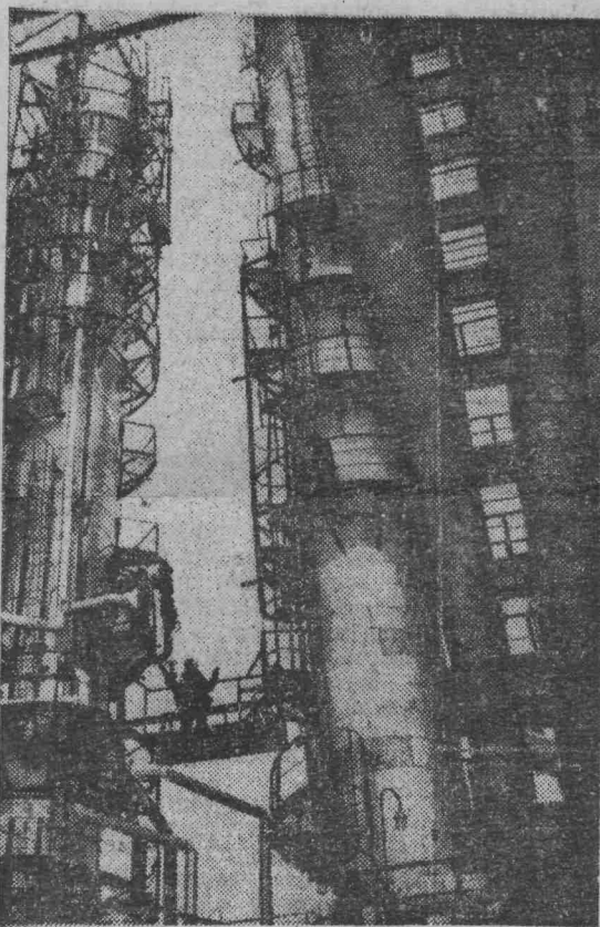
Получены первые тонны бензина на новой атмосферно-вакуумной трубчатке Ново-Ярославского нефтеперерабатывающего завода.
