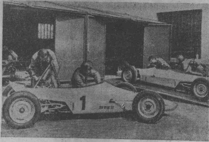
НА ОДНОМ из предприятий в городе Пльзень выпущена серия гоночных автомашин «Шкода» МТХ. Новые автомобили имеют ряд преимуществ по сравнению с ранее выпускаемыми моделями. Машина, построенная на базе деталей и агрегатов широко распространенных малолитражек «Шкода 100» и «Шкода 110», имеет так называемый «скоростной» кузов и регулируемые по росту водителя педаль и рулевое колесо.
