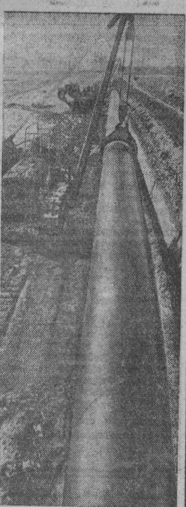
Челябинская область. Этот снимок сделан на одном из участков строительства трансконтинентального нефтепровода Усть-Балык—Курган—Уфа—Альметьевск, которое ведут тресты «Уралнефтегазстрой», «Нефтепроводмонтаж» и ряд других организаций. С вводом его в действие сибирская нефть получит выход не только на перерабатывающие заводы Поволжья, но и через систему «Дружба» — в социалистические страны Европы.
