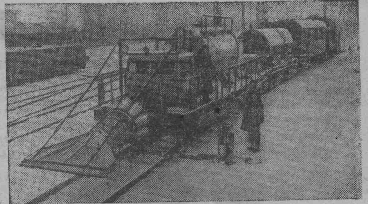
При заносах на железнодорожных путях Будапешта для очистки стрелок от снега используется специальное устройство. Выработываемый им газ горячей струей подается на рельсы, вызывая таяние снежного покрова. За час машина обрабатывает таким образом 25—28 стрелок.
