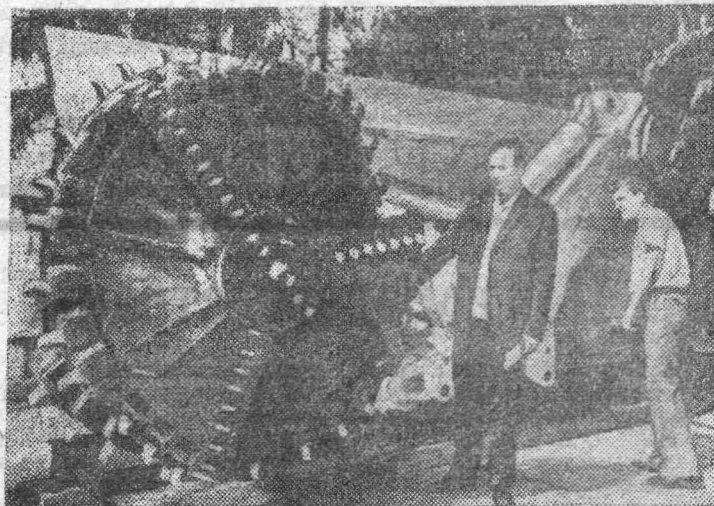
Москва. На ВДНХ СССР в павильоне «Угольная промышленность» демонстрируется очистной узкозахватный комбайн КПШ-3М. Он предназначен для выемки угля из пластов мощностью 1,8—3,3 метра с углом падения до 20 градусов. Комбайн, изготовленный на Горловском машиностроительном заводе имени С. М. Кирова и на экспериментальном заводе Подмоск. научно-исследовательского и проектно-конструкторского угольного института, снабжен средствами пылеподавления: оросительными и пылеотсасывающими устройствами.
