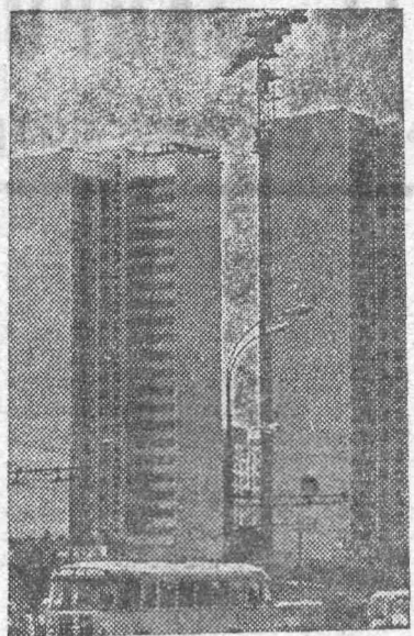
Москва. Строительно-монтажное управление СКБ «Прокатдеталь» возводит в Тропареве три экспериментальных двадцатидвухэтажных жилых дома. В каждом из них по 147 двух-, трех- и четырехкомнатных квартир улучшенной планировки. Монтаж жилых домов ведется из унифицированных деталей по единому каталогу. На снимке: строительство экспериментальных зданий в Тропареве. Фото В. Кошевого. (Фотохроника ТАСС).
