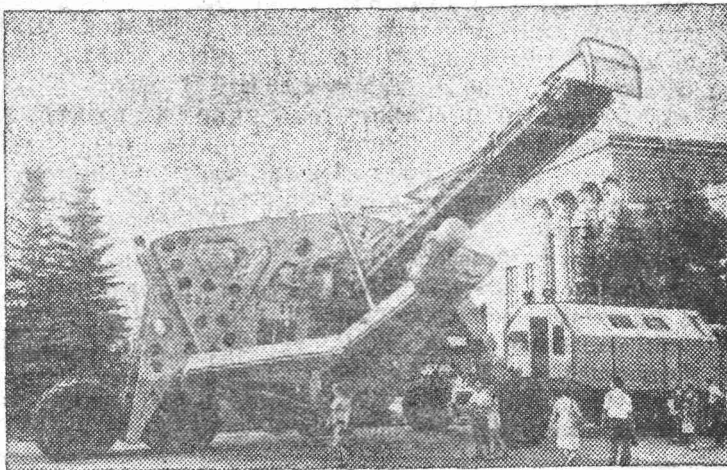
МОСКВА. На ВДНХ СССР демонстрируется гигантский шнекороторный экскаватор ЭТР-301, предназначенный для прокладки ирригационных каналов глубиной до 3 метров и шириной по дну до 2,5 метра. Производительность машины — 400 кубических метров в час. Обслуживающий персонал — 3 человека.
