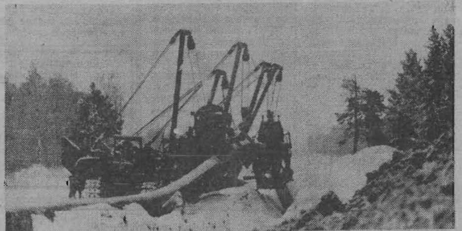
На снимках: машинист трубоукладчика Виктор Горбанев; строительство газопровода в районе Кривопольца (Томская область) велет производственное объединение «Южгаспромстрой» из Ростова-на-Дону. Фото Ю. Дьячкова. Творческая студия «Панорама».
