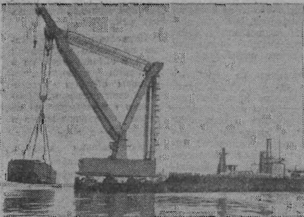
На снимке: идут испытания крана. Его 79-метровая стрела подняла понтон, наполненный водой, весом в тысячу тонн. Фото В. Пащенко. (Фотохроника ТАСС).
