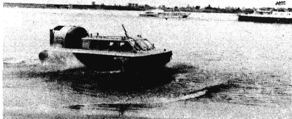
Коллектив конструкторского бюро производственного объединения «Завод «Красное Сормово» впервые на таком типе судов применил в качестве силовой установки дизельный двигатель.
