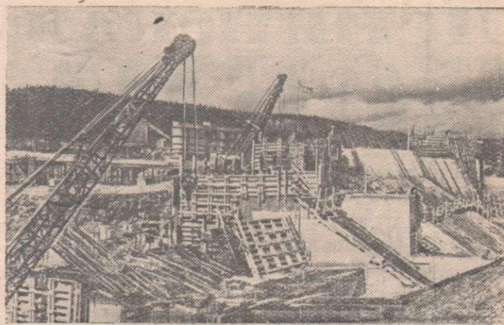
Башкирская АССР. На строительстве Уфимской ГЭС.
