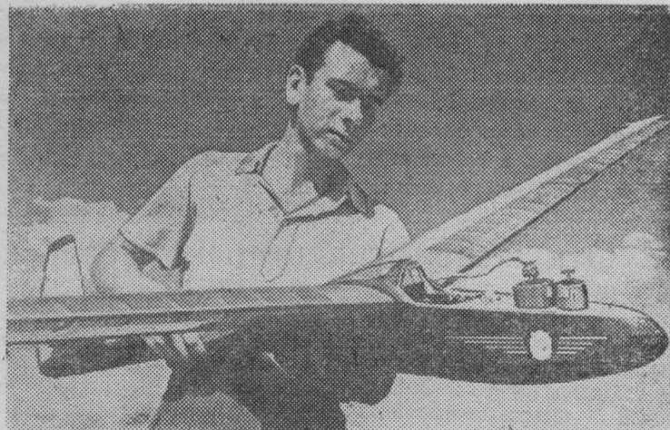
Украинская ССР. Студент 3-го курса Харьковского авиационного института комсомолец Владимир Орехов установил Всесоюзный и мировой рекорд на дальность полета модели планера, управляемого по радио. Пробыв в воздухе 28 минут 15 секунд, модель пролетела по прямой 3680 метров.
