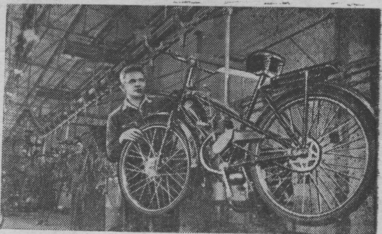
Львов. Мотовелосипеды «В-902», выпускаемые заводом «Металл» очень удобная дорожная машина, способная нести на себе груз до 100 кг и развивать скорость до 45 км в час. Предприятие ежемесячно выпускает до 6.500 мотовелосипедов. На снимке: сборка мотовелосипедов на конвейере. Фото К. Бузынина. Фотохроника ТАСС
